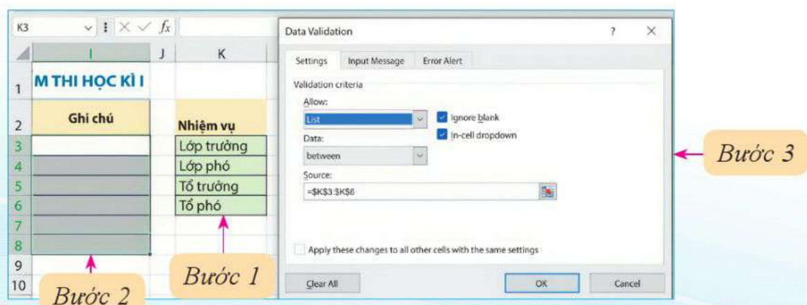
Hình 3. Ví dụ thiết lập nhập dữ liệu cho cột Ghi chú bằng danh sách
