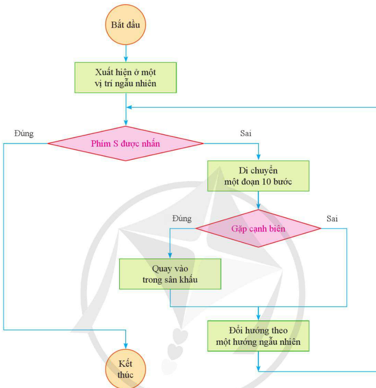
Hình 5. Một mô tả thuật toán điều khiển bóng hồng bằng sơ đồ khối
