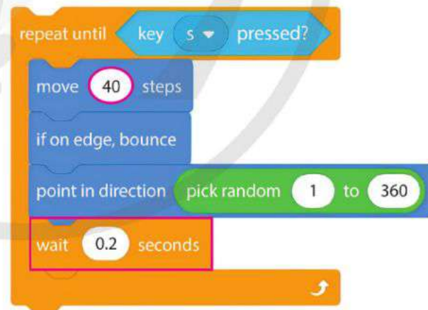
Hình 6. Một điều chỉnh trong chương trình điều khiển bóng hồng
