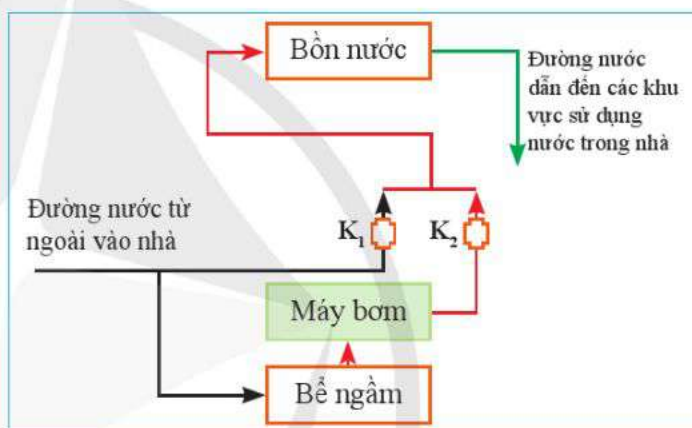
Hình 4. Một hệ thống đường nước trong nhà
