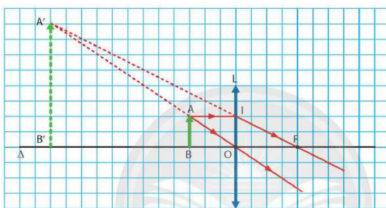
▲ Hình 7.13. Sơ đồ tỉ lệ tạo ảnh ảo của vật qua thấu kính hội tụ
