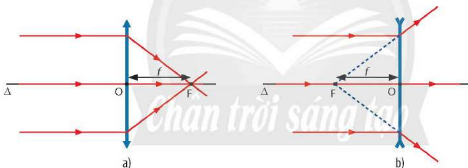
▲ Hình 7.6. Sơ đồ đường đi của các tia sáng song song qua: a) thấu kính hội tụ; b) thấu kính phân kì
