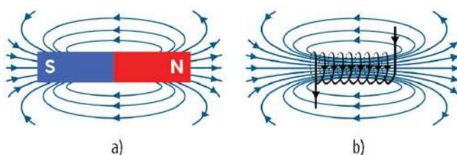
▲ Hình 12.3. Các đường sức từ của: a) nam châm thẳng; b) nam châm điện (ống dây mang dòng điện)
