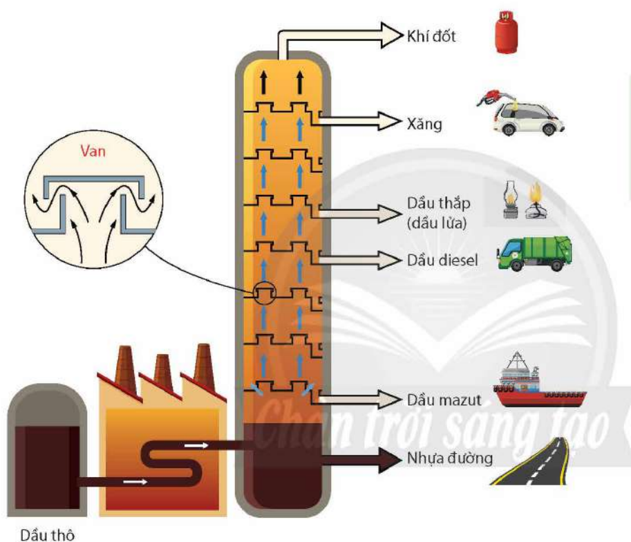
▲ Hình 23.2. Mô hình tháp chưng cất dầu thô
