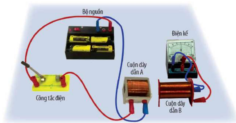
▲ Hình 12.2. Bố trí thí nghiệm dùng nam châm điện để tạo ra dòng điện
